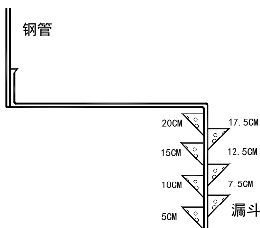
图 4 Z 字型量泥斗构造图
