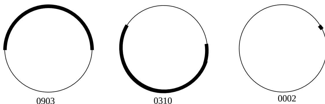
图1 缺陷环向位置时钟表示法示例
