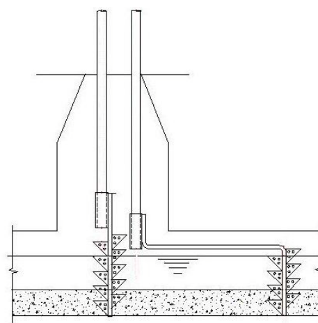
图 5 量泥斗检查示意图
