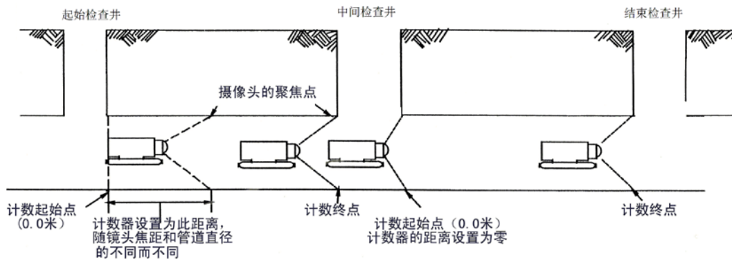
图 2 计数器归零的补偿设置方法示意图
