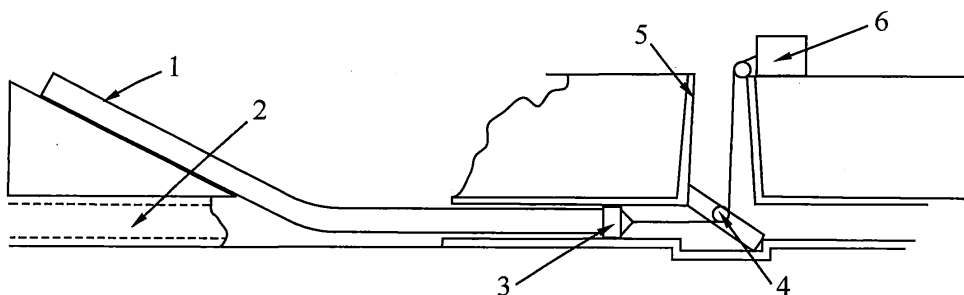
图 1 连续管道穿插法示意图
